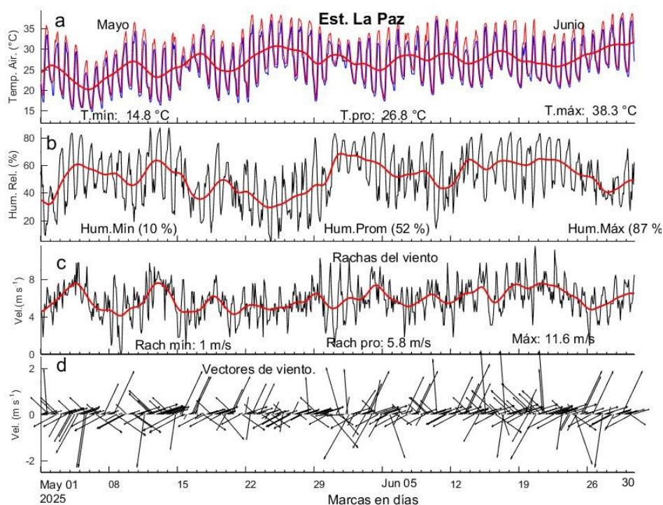
Figura 7.1: Series de tiempo de variables atmosféricas registradas en la Estación La Paz, desde el 01 de mayo al 30 de junio): (a) Temperatura del aire máxima (rojo) y mínimas (azul), (b) Humedad Relativa, (c) Rachas del viento y (d) la dirección del vector del viento (de donde viene el viento). Las líneas en rojo indican las series suavizadas a partir del promedio corrido de 24 hrs., de cada variable analizada.
