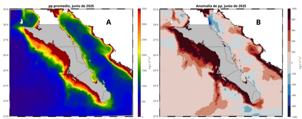
Figura 3.2: Condiciones de PPN durante el mes de junio de 2025. Panel A, condiciones mensuales promedio y panel B, anomalías mensuales.
