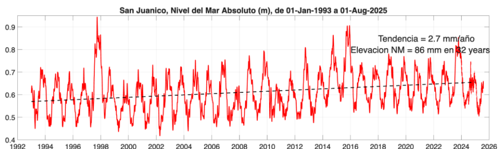
Figura 2.5: Nivel del mar absoluto (m) en la San Juanico, BCS, costa pacífico norte de BCS. Inicia en enero de 1993 y termina en julio de 2025. Incluye el nivel del mar con referencia al geoides y la tendencia de largo período debida al calentamiento global. Este sitio representa la variabilidad del Golfo de Ulloa.
