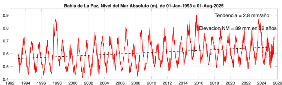
Figura 2.4: Nivel del mar absoluto (m) en la bahía de La Paz, BCS. Inicia en enero de 1993 y termina en julio de 2025. Incluye el nivel del mar con referencia al geoides y la tendencia de largo período debida al calentamiento global.
