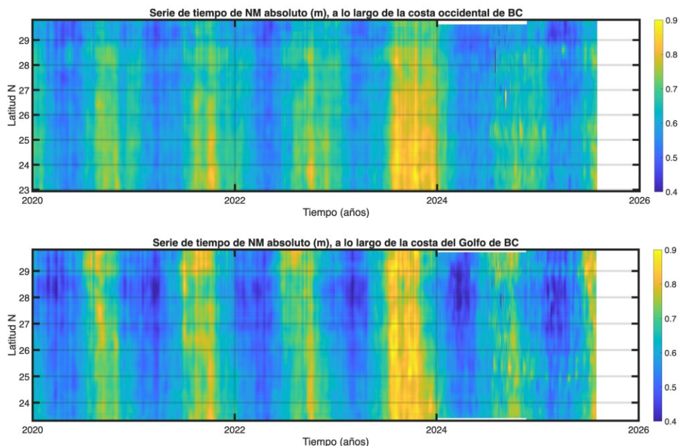
Figura 2.2: Los últimos años de la evolución del nivel del mar (NM absoluto) a lo largo de las dos costas de la península de BC desde enero de 2020 hasta julio de 2025. Arriba: costa
