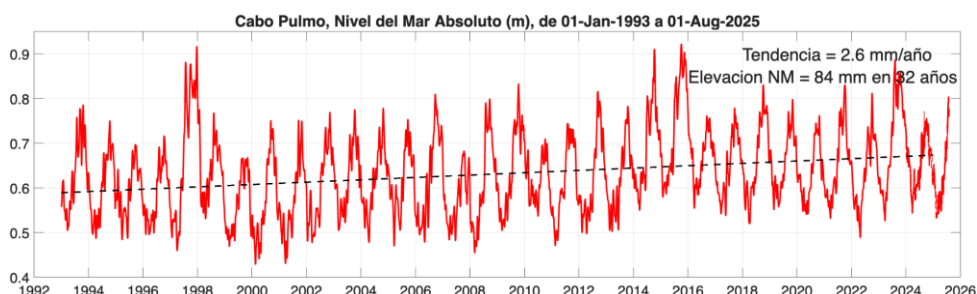
Figura 2.3: Nivel del mar absoluto (m) en Cabo Pulmo, BCS. Inicia en enero de 1993 y termina en julio de 2025. Incluye el nivel del mar con referencia al geoide y la tendencia de largo período debida al calentamiento global. Este sitio representa la variabilidad de la entrada al Golfo de California.
