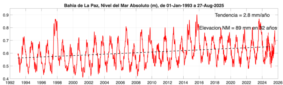
Figura 2.4: Nivel del mar absoluto (m) en la bahía de La Paz, BCS. Inicia en enero de 1993 y termina en agosto de 2025. Incluye el nivel del mar con referencia al geoido y la tendencia de largo período debida al calentamiento global.
