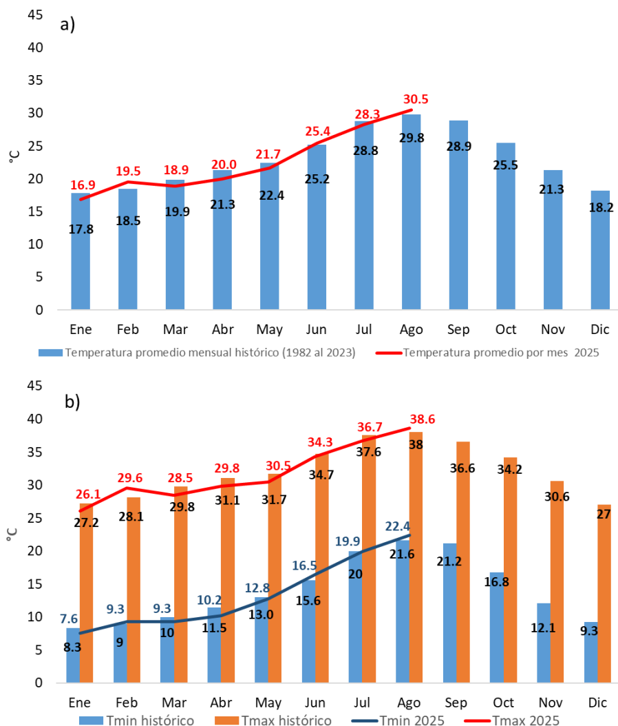
Figura 8.2: a) Comparativo de los promedios mensuales de la temperatura media (periodo 1982-2023) con respecto al registrado al mes de agosto de 2025. b) Comparativo entre los promedios de temperaturas máximas y mínimas históricas (1982-2023) con respecto a los promedios presentados al mes de agosto de 2025. Tmax= Temperatura máxima. Tmin= Temperatura mínima.
