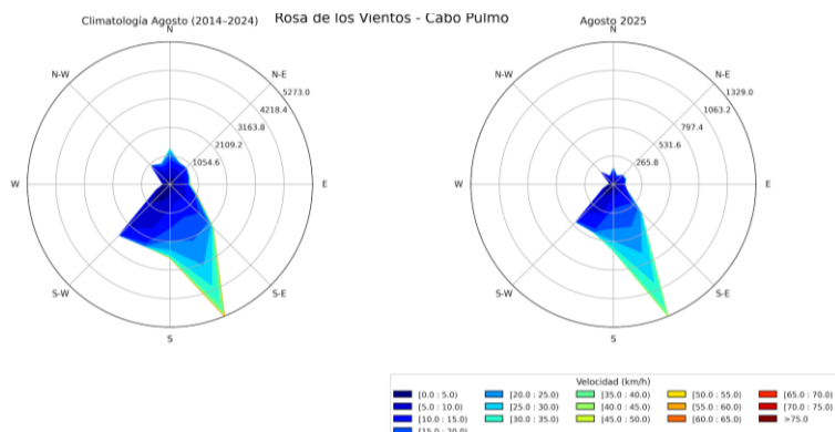
Figura 6.1: Climatología vs. observaciones de la dirección e intensidad de los vientos en la estación Cabo Pulmo durante el mes de agosto de 2025.
