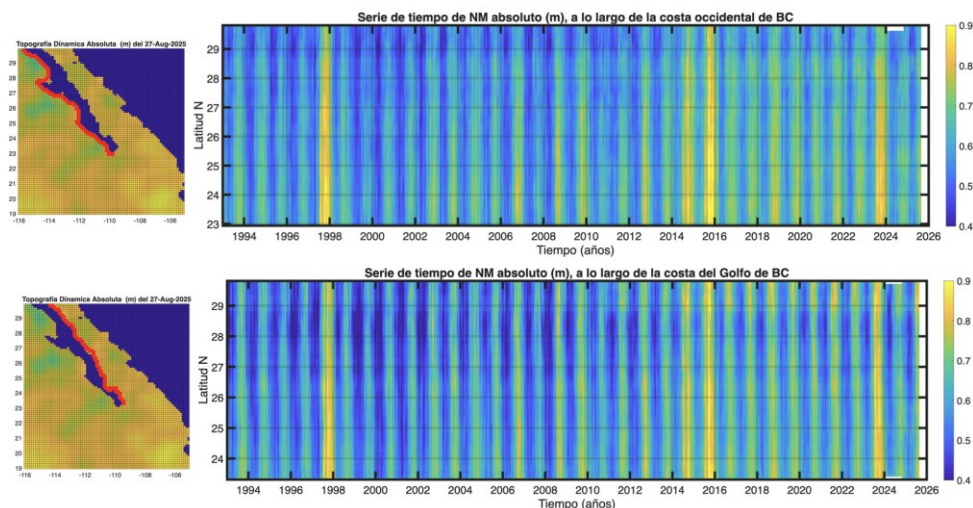
Figura 2.1: Evolución del nivel del mar (NM absoluto) a lo largo de las dos costas de la península de BC desde enero de 1993 hasta agosto de 2025. Arriba: costa occidental; abajo: costa del Golfo de California.
