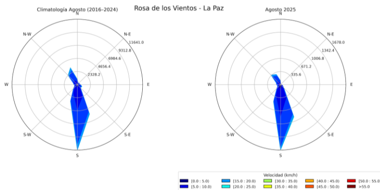
Figura 6.3: Climatología vs. observaciones de la dirección e intensidad de los vientos en la estación ESIME de La Paz durante agosto de 2025.
