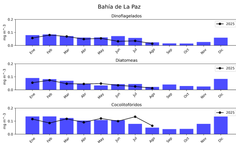
Figura 5.2: Estas climatologías representan la concentración de grupos fitoplanctónicos, expresada en CLO en el agua de mar en la bahía de La Paz durante agosto de 2025. La concentración de los grupos fitoplanctónicos se muestra como una representación visual de la información estimada por el modelo PHYSAT de COPERNICUS.
