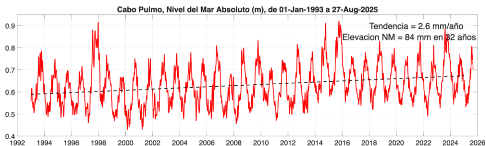
Figura 2.3: Nivel del mar absoluto (m) en Cabo Pulmo, BCS. Inicia en enero de 1993 y termina en agosto de 2025. Incluye el nivel del mar con referencia al geoide y la tendencia de largo período debida al calentamiento global. Este sitio representa la variabilidad de la entrada al Golfo de California.
