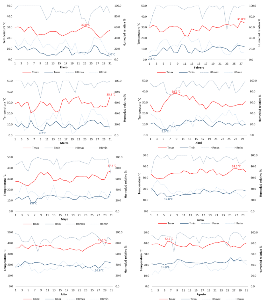
Figura 8.1: Comportamiento de la temperatura y humedad relativa al mes de agosto de 2025. Tmax= Temperatura máxima. Tmin= Temperatura mínima. HRmax= Humedad relativa máxima. HRmin= Humedad relativa mínima. Los valores en rojo y azul dentro de cada mes, indican el valor más alto y el más bajo de las temperaturas máxima y mínima, respectivamente.
