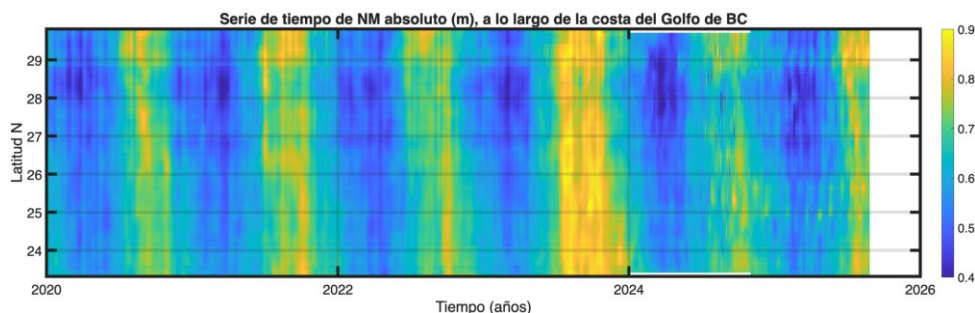
Figura 2.2: Los últimos años de la evolución del nivel del mar (NM absoluto) a lo largo de las dos costas de la península de BC desde enero de 2020 hasta agosto de 2025. Arriba: costa occidental; abajo: costa del Golfo de California.
