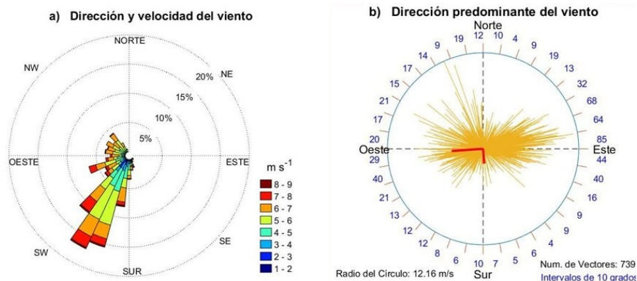
Figura 7.2: Velocidad y dirección (16 direcciones) del viento registradas durante el período de julio-agosto, 2025 (verano) en la BLPZ graficados como: a) Rosa del viento (dirección y velocidad) y (b) vectores del viento que indica la frecuencia y el número de vectores calculados (cada 10 grados). Los vectores en rojo indican los ejes principales promedio de la máxima y mínima varianza de La dirección del viento registrado durante el período analizado.
