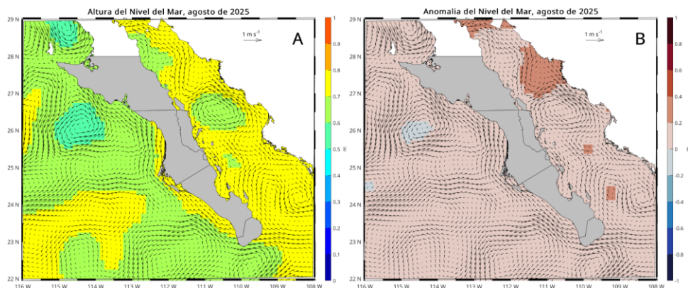
Figura 3.3: Condiciones mensuales de altimetría durante el mes de agosto de 2025. Panel A, altura del mar (ADT) promedio y panel B, anomalías del nivel del mar (SLA), en ambos casos con el promedio mensual de las corrientes geostróficas (CORR) superpuestas en forma de flechas.
