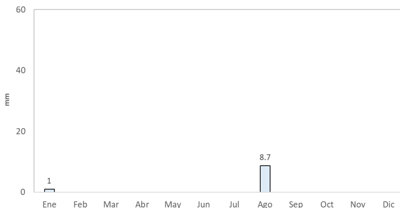
Figura 8.4: Precipitación acumulada por mes hasta agosto de 2025.
