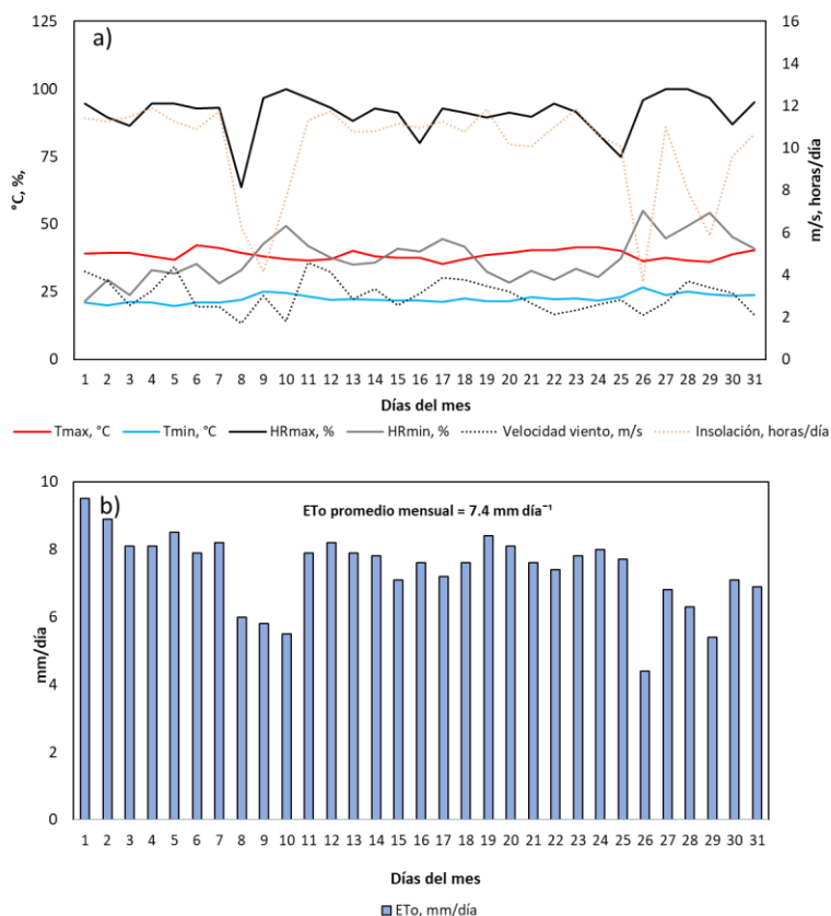
Figura 8.3: a) Comportamiento de la temperatura máxima (Tmax), temperatura mínima (Tmin), humedad relativa máxima (HRmax) y mínima (HRmin), velocidad del viento e insolación en el mes de agosto de 2025. b) Comportamiento de la evapotranspiración potencial (ETo) para el mes de agosto de 2025.
