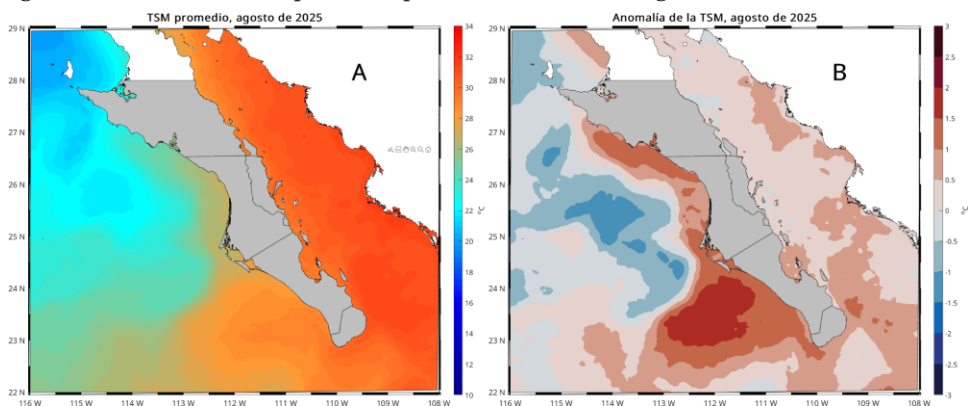
Figura 3.1. Condiciones mensuales de TSM durante el mes de agosto de 2025. Panel A, promedio y panel B, anomalías.
