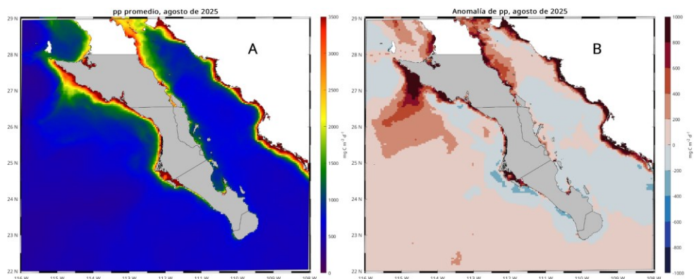
Figura 3.2: Condiciones mensuales de PP durante el mes de agosto de 2025. Panel A, condiciones promedio y panel B, anomalías.
