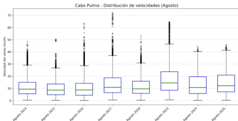
Figura 6.2: Análisis de cajas de la intensidad de los vientos en la estación Cabo Pulmo durante el mes de agosto de 2025. Los valores de viento atípico están dados en el gráfico de cajas por los outliers (círculos en negro).
