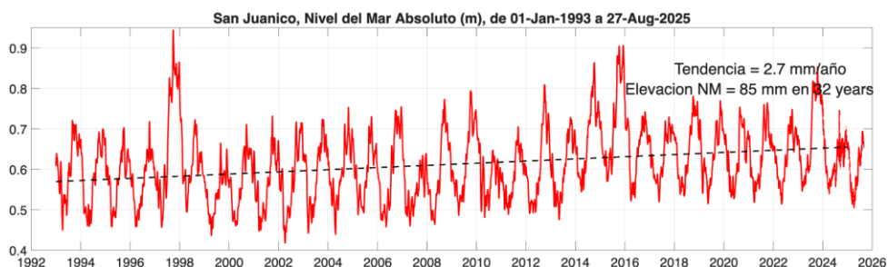
Figura 2.5: Nivel del mar absoluto (m) en la San Juanico, BCS, costa pacífico norte de BCS. Inicia en enero de 1993 y termina en agosto de 2025. Incluye el nivel del mar con referencia al geode y la tendencia de largo período debida al calentamiento global. Este sitio representa la variabilidad del Golfo de Ulloa.
