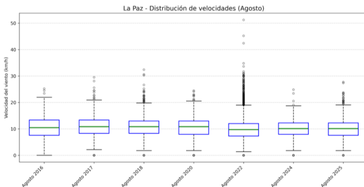
Figura 6.4: Análisis de cajas de la intensidad de los vientos en la ciudad de La Paz, BCS, durante el mes de agosto de 2025. Los valores de viento atípico u outliers se muestran con círculos en negro en la figura.
