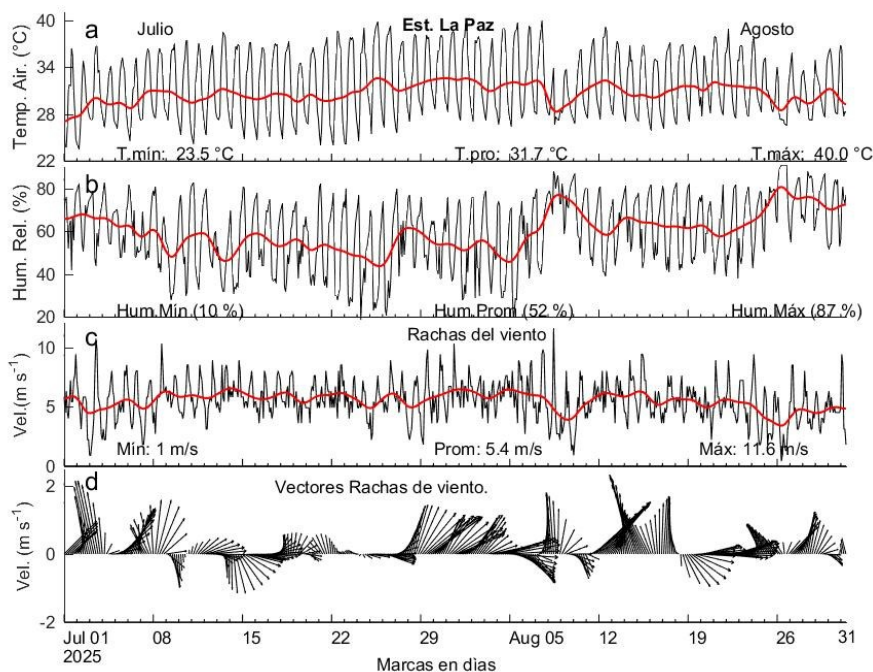
Figura 7.1: Series de tiempo de variables atmosféricas registradas en la Estación La Paz, desde el 01 de julio al 31 de agosto: (a) Temperatura del aire máximas (en negro), (b) Humedad Relativa, (c) Rachas del viento y (d) la dirección del vector del viento (de donde viene el viento). Las líneas en rojo indican las series suavizadas a partir del promedio corrido de 24 hrs., de cada variable analizada.
